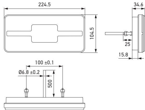
Maßskizze
