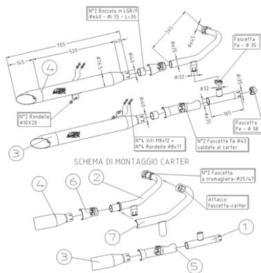
ART.2244 YAMAHA XVS 1100 DRAG STAR Silenziali <<AD2>> OMOLOGATO
